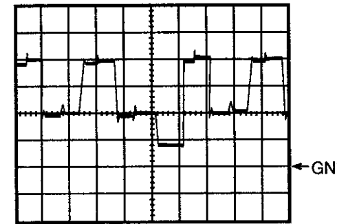
WF15 1DIV: 2V 10 μsec
