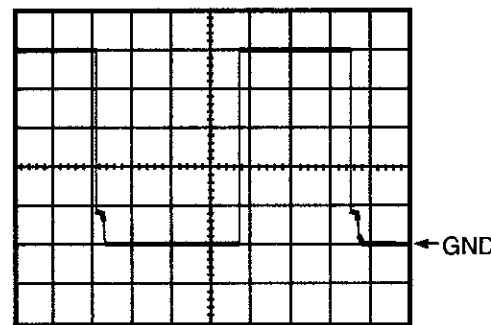
WF7 1DIV: 1V 10 μsec
