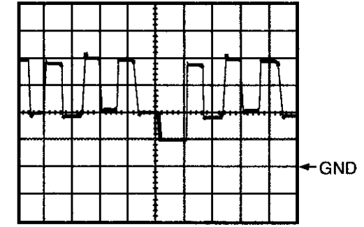
WF17 1DIV: 2V 10 μsec
